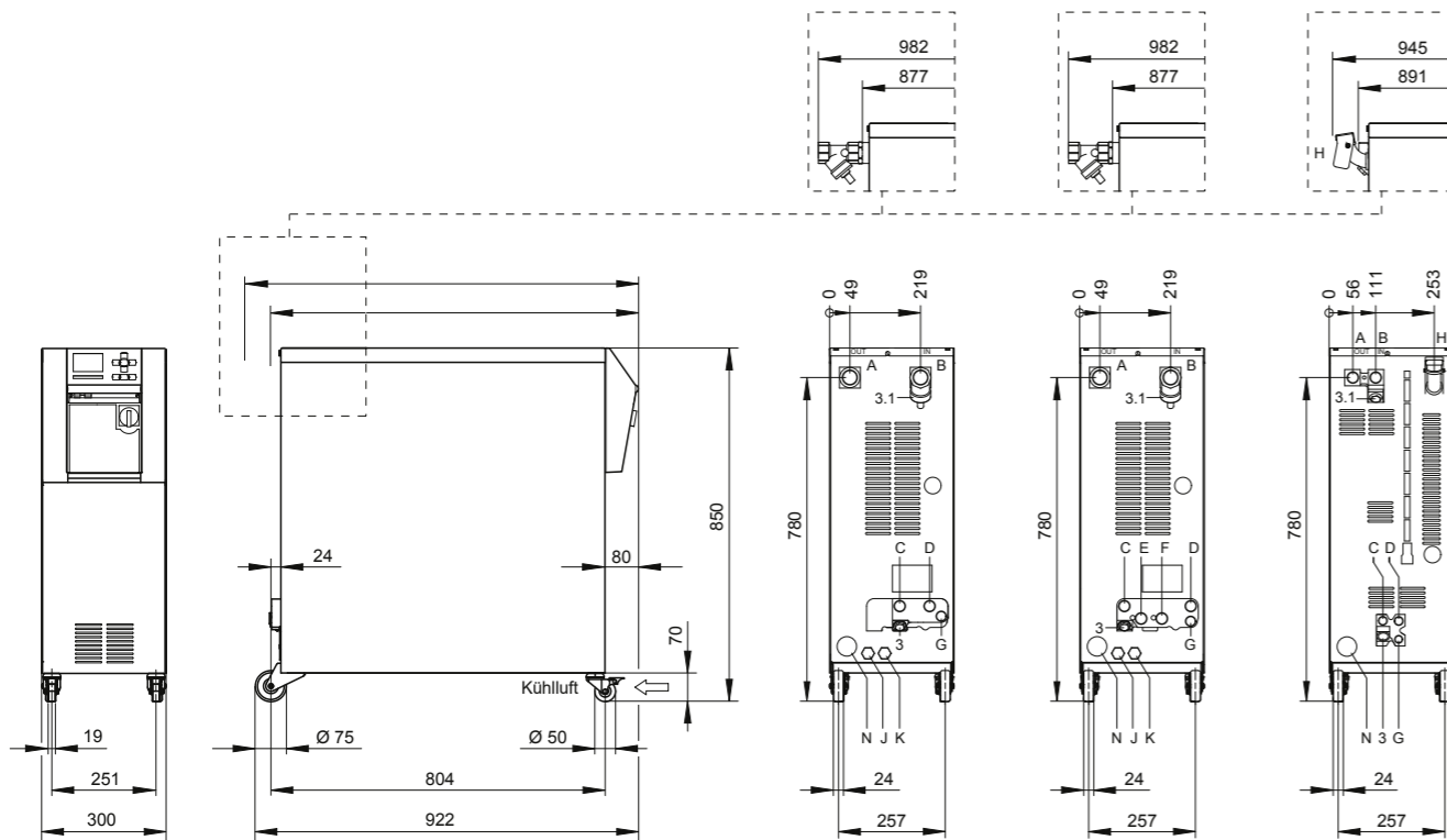
Baugröße 3, Massstab 1:20
