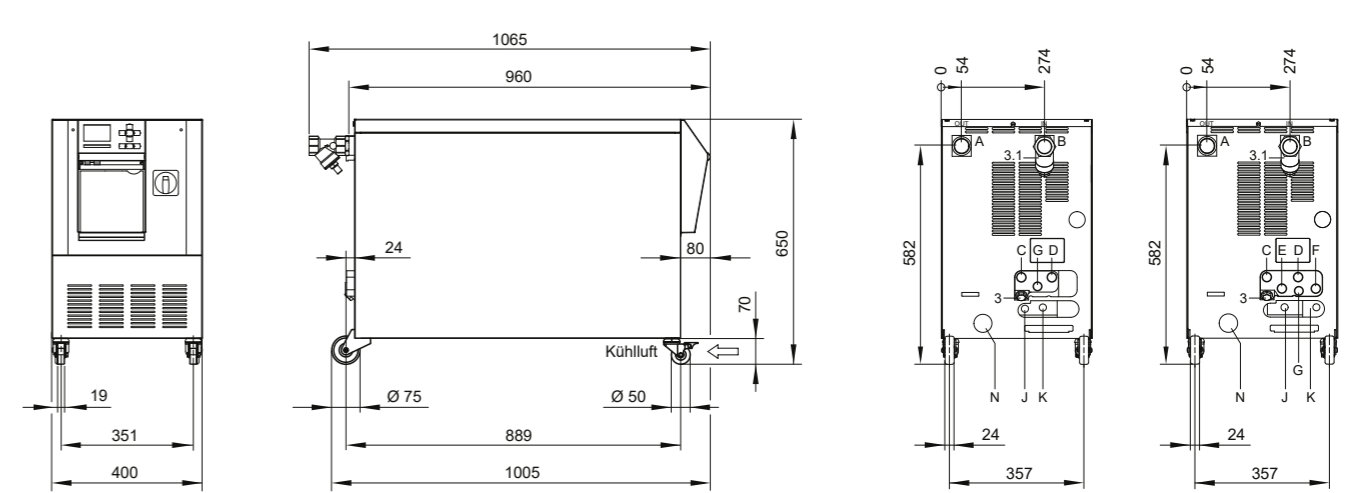
Baugröße 4, Massstab 1:20
